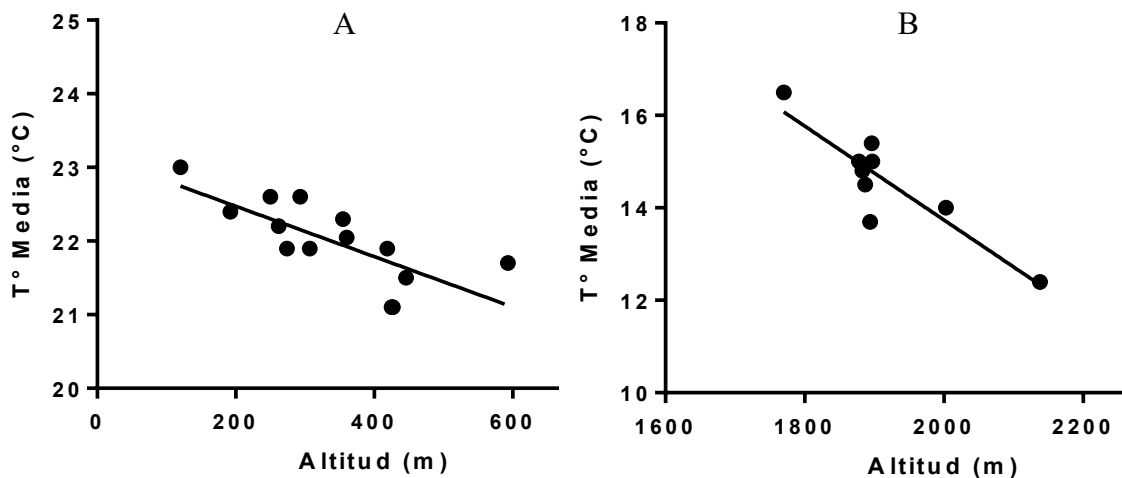
Fig. 2. Modelos de regresión entre la altitud y temperatura media. A: Región baja; B: Región alta
