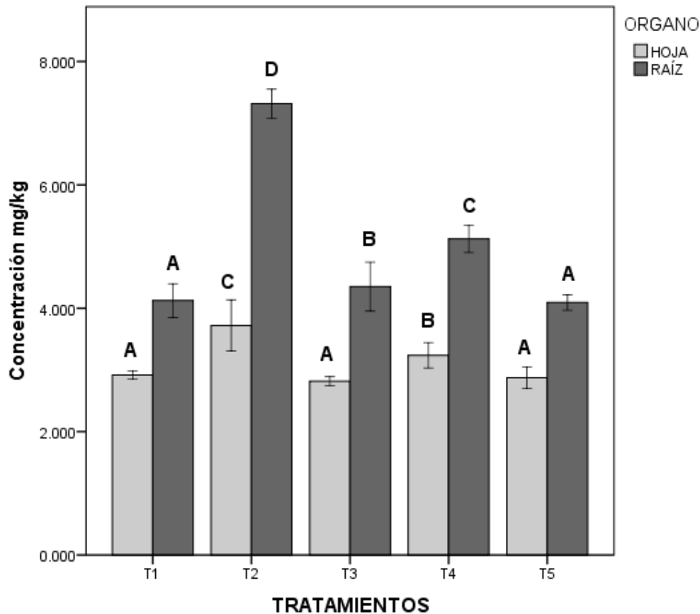
Figura 5. Concentración de Vanadio en Chrysopogon zizanioides . Medias de órganos por tratamiento con una letra común no son significativamente diferentes ( p > 0.05 ).
