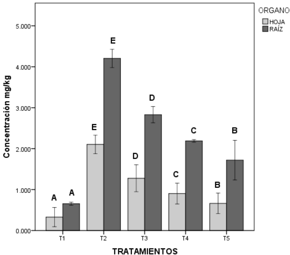
Figura 4. Concentración de Plomo en Chrysopogon zizanioides .
